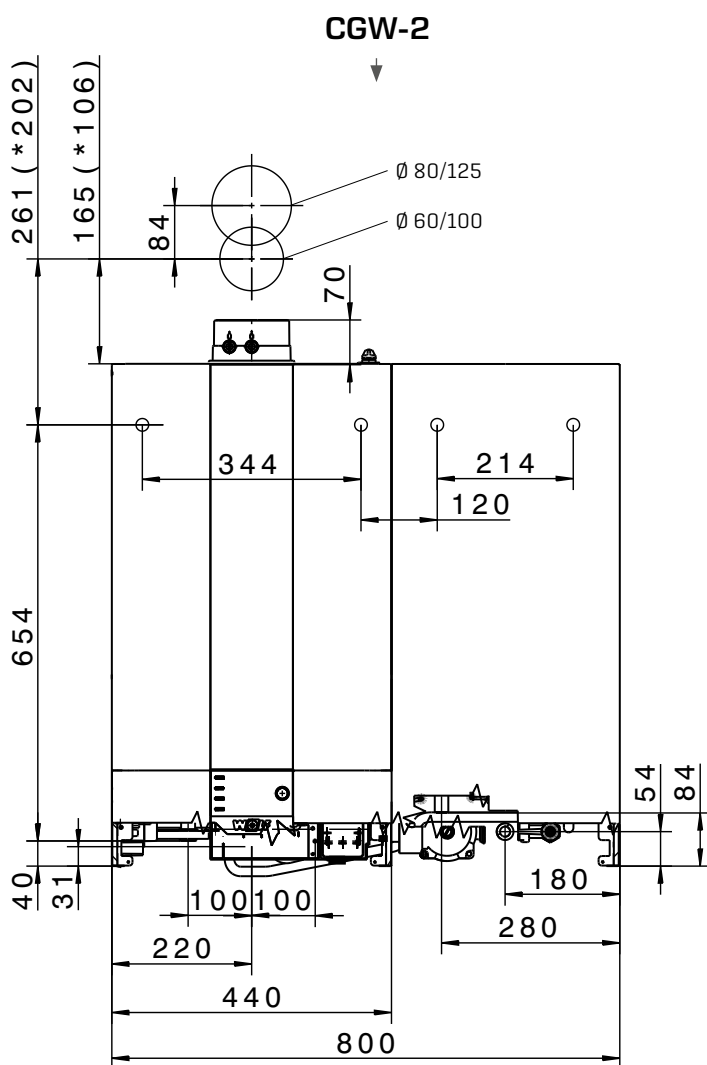
Вид спереди
